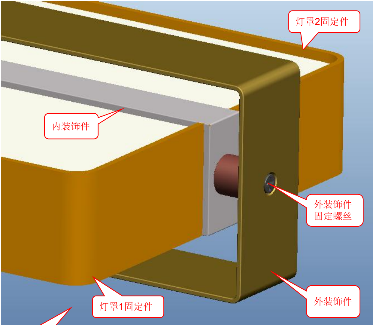
侧面视图
