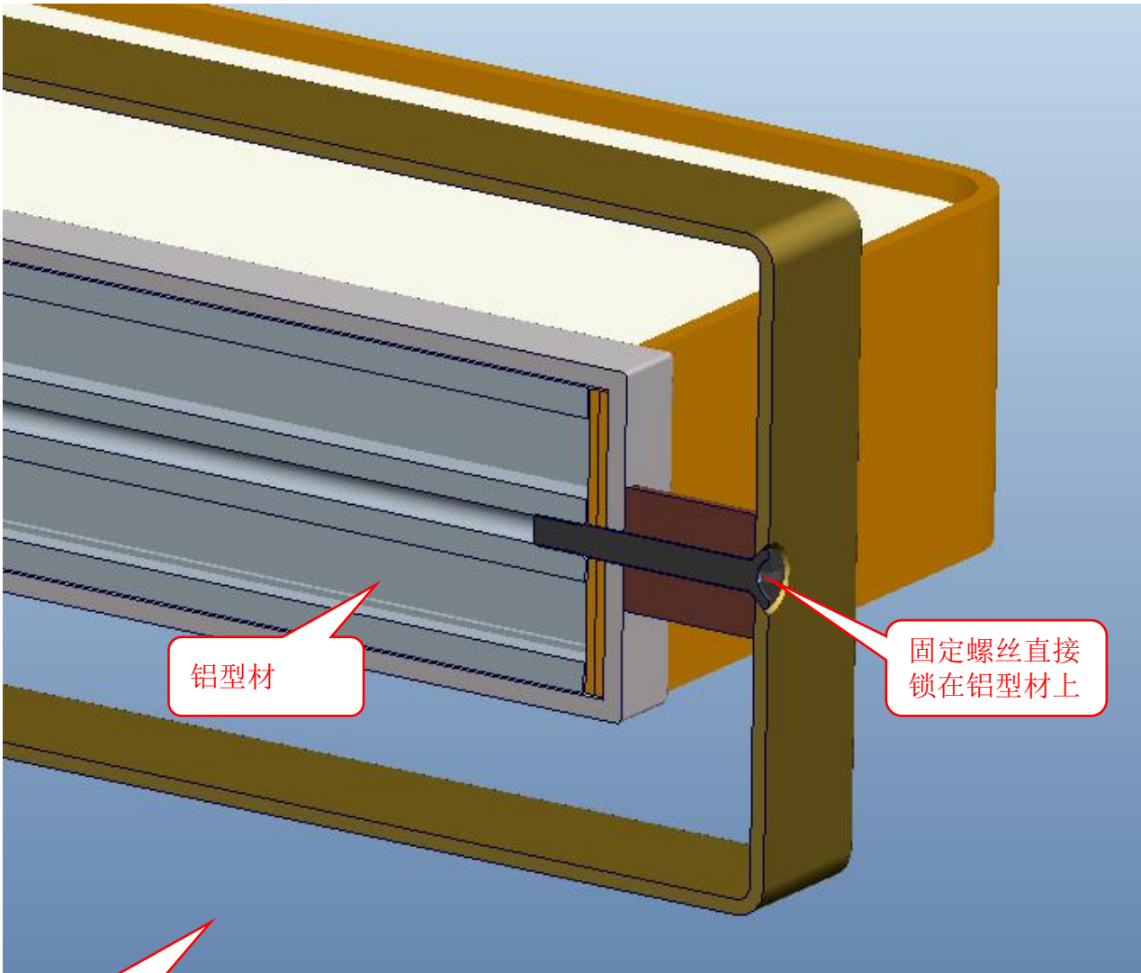
剖面图
